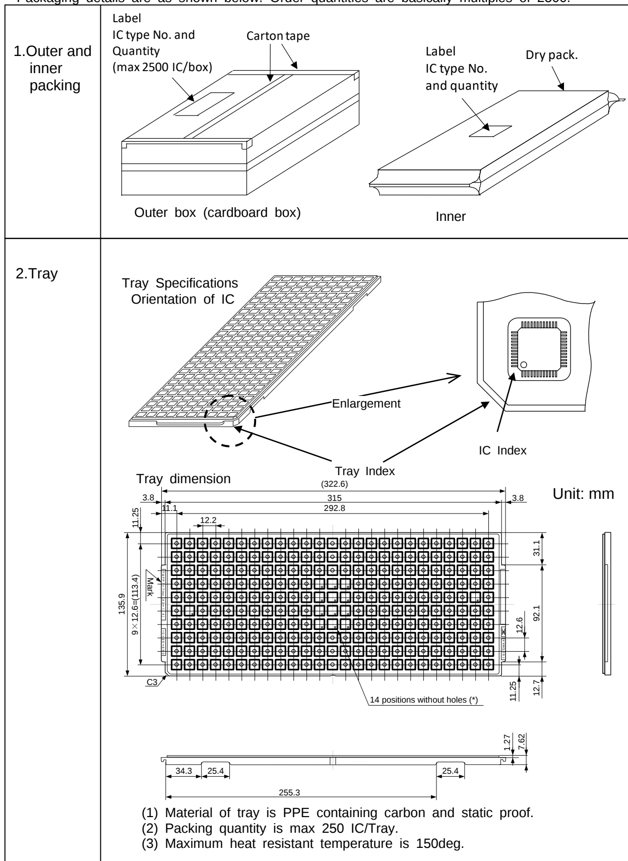
Fig.C IC packing det
