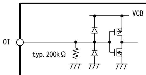
図2.2.5 OT端子の等価回路
