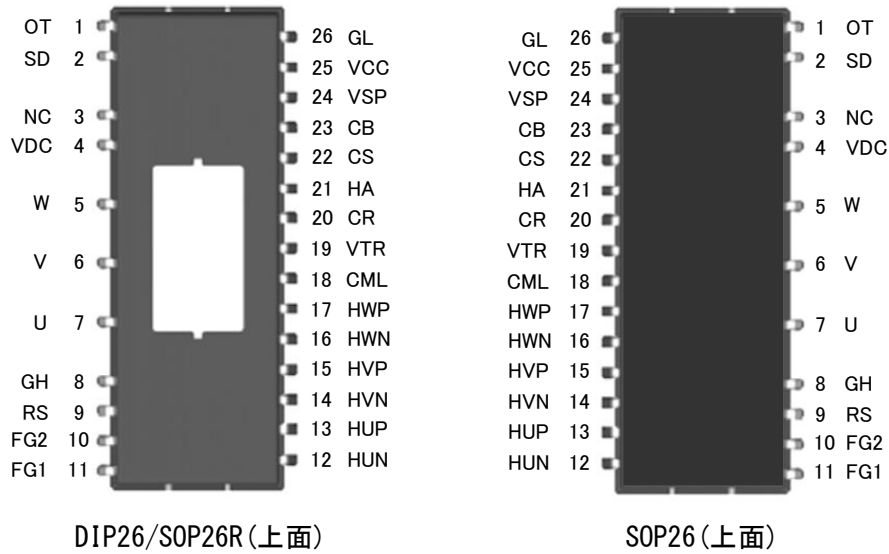
図5.1 端子配置
