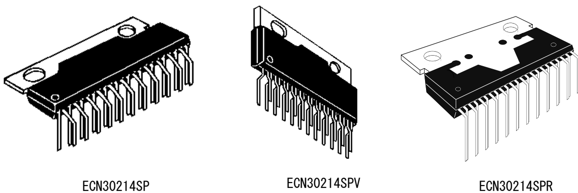
図1.4.1 ECN30214の外形
