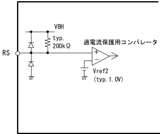
図 2.2.1 RS 端子の等価回路
