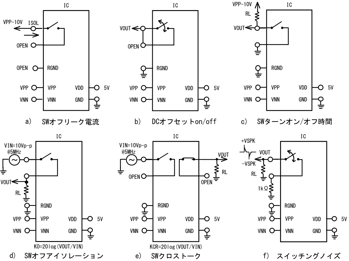
図 4.1 測定回路
