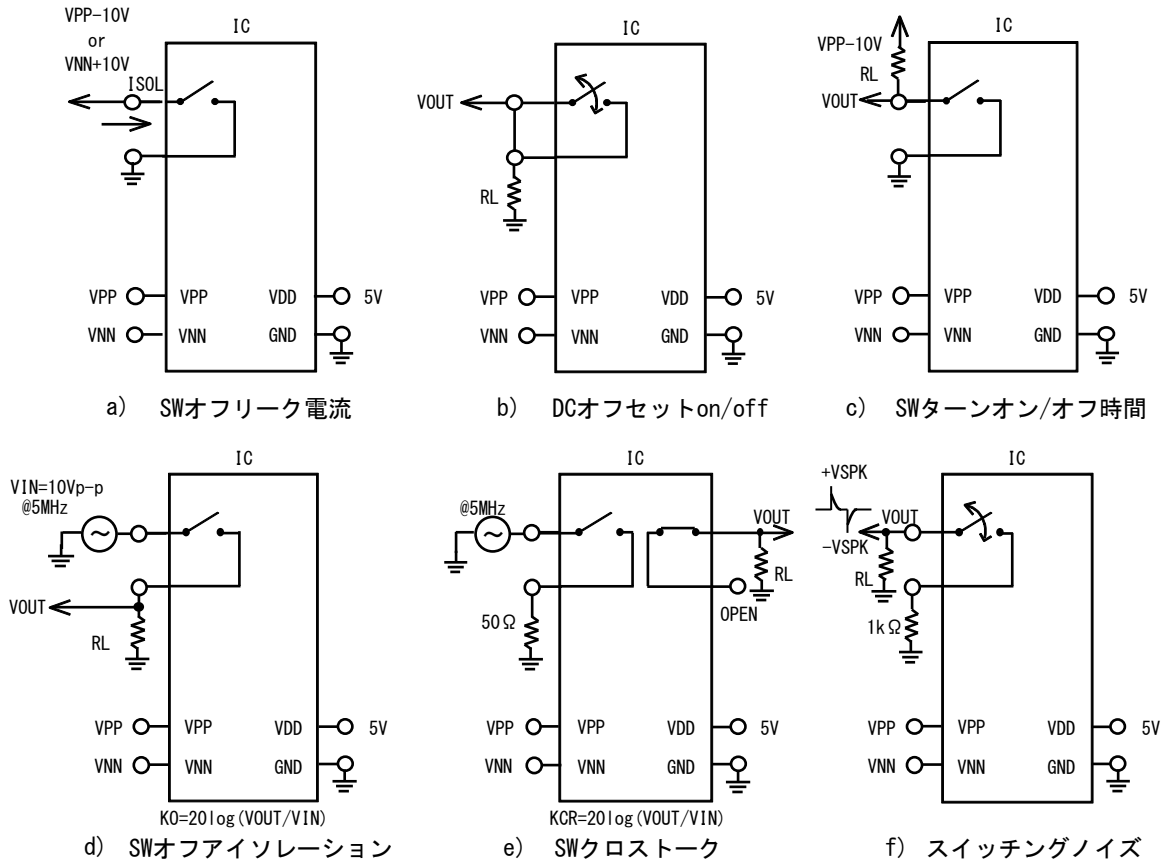
図 4.1 測定回路
