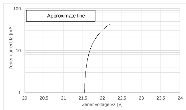
Fig.A-6. Zener current – Zener voltage *
