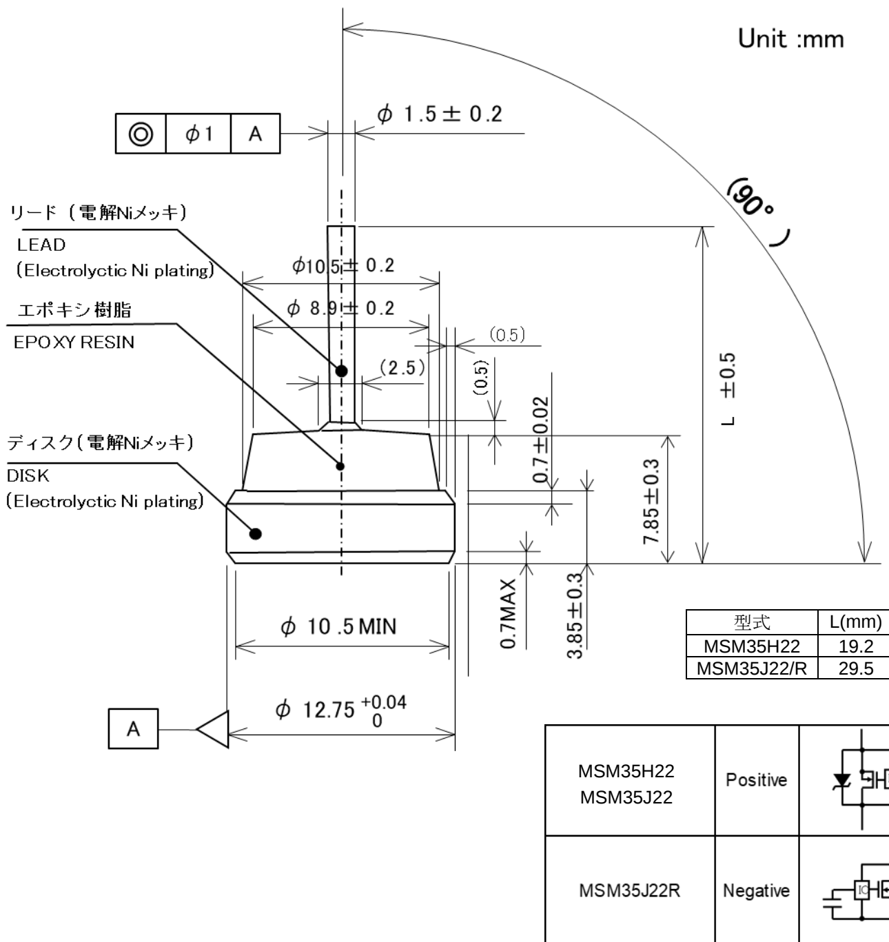
Fig 5. Physical Dimensions 外形寸法
