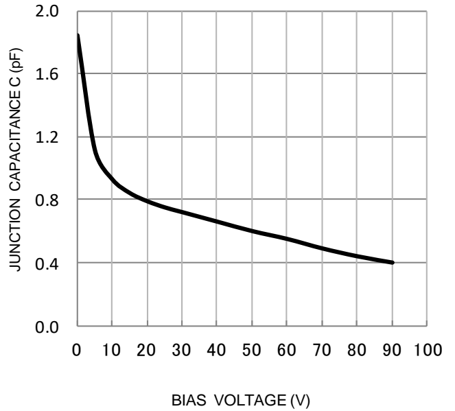
逆特性 (代表例)
