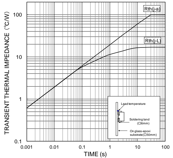
過渡熱インピーダンス
